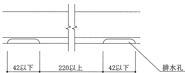
背面図
